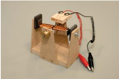
Construcció d'un motor de corrent continu
