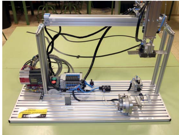
Estació de treball programable
