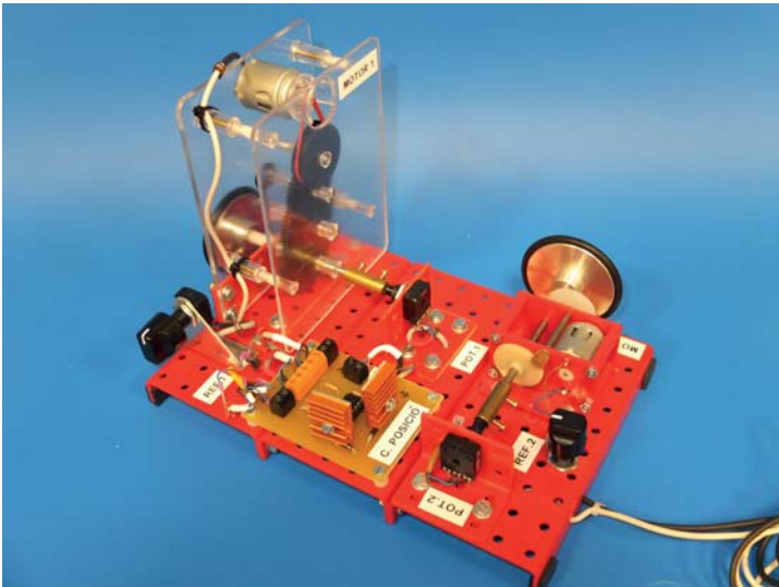
Servosistema: seguidor de posició
